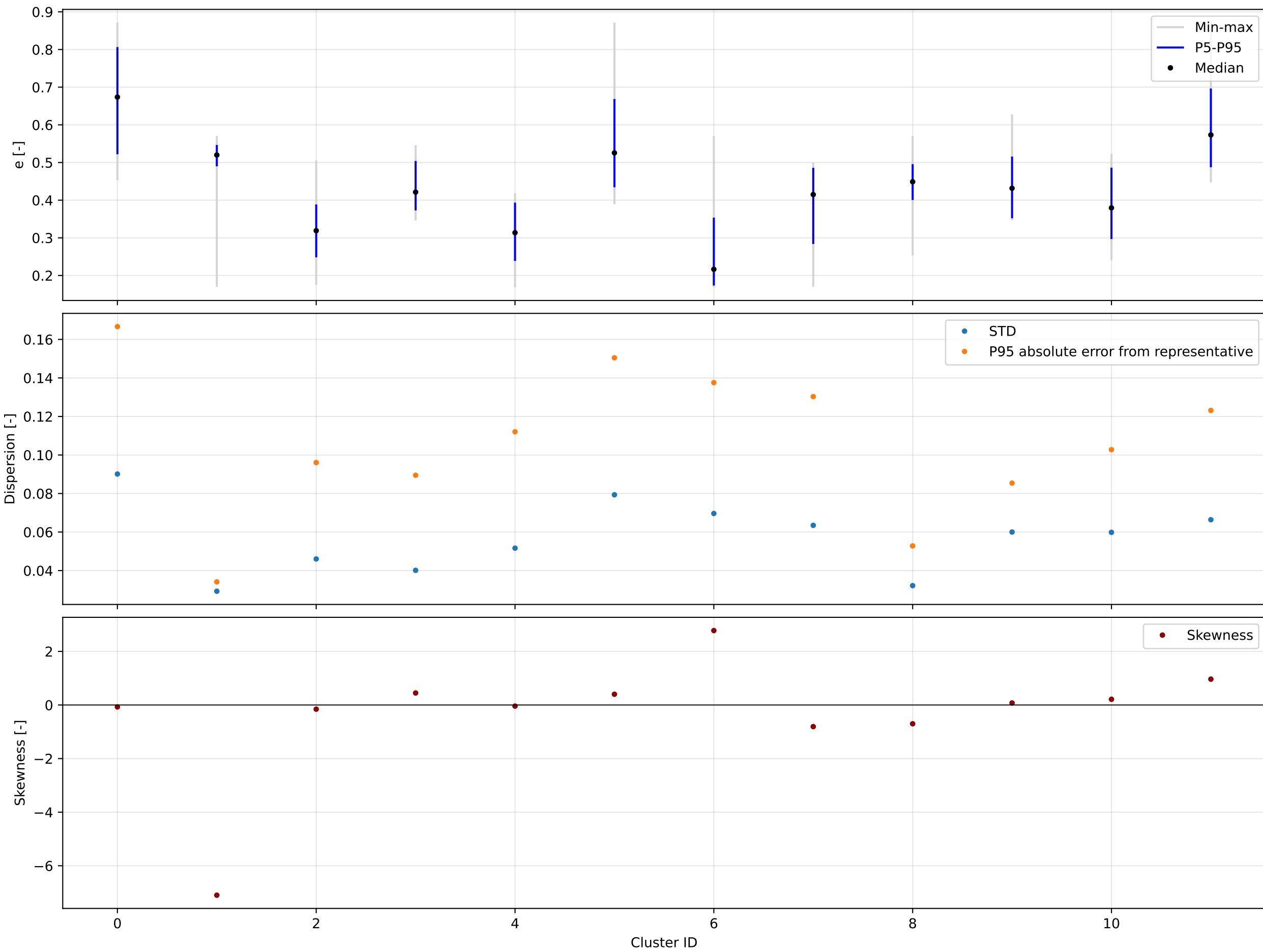
K=12 | backward | e | valid=194058/194058
